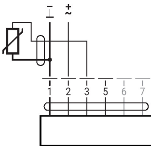
Anschluss mit passivem Sensor
