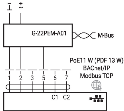
Anschluss mit aktivem Sensor
