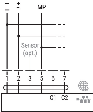
M-Bus mit Konverter im Parallelbetrieb mit BACnet/IP / Modbus TCP
