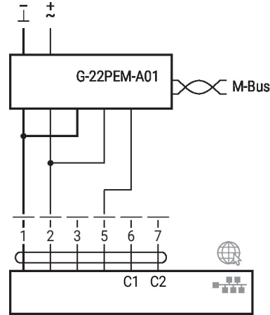
M-Bus mit Konverter im Parallelbetrieb mit PoE mit BACnet/IP / Modbus TCP
