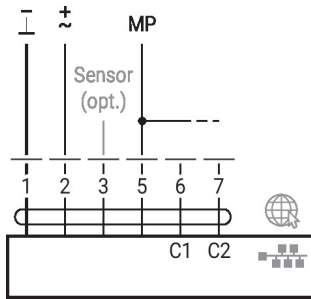
M-Bus mit Konverter im Parallelbetrieb mit BACnet/IP / Modbus TCP
